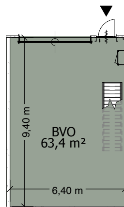
BEGANE GROND
